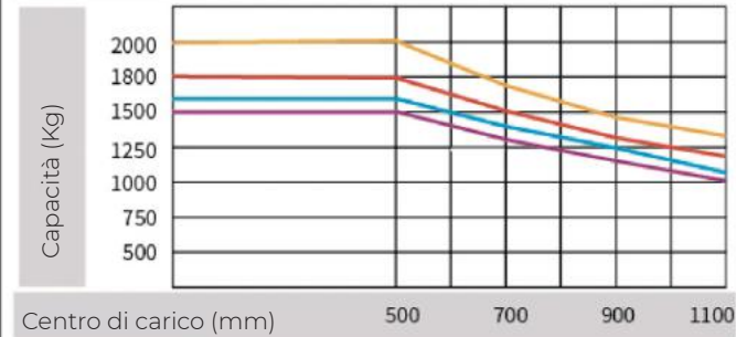
Curva di carico
